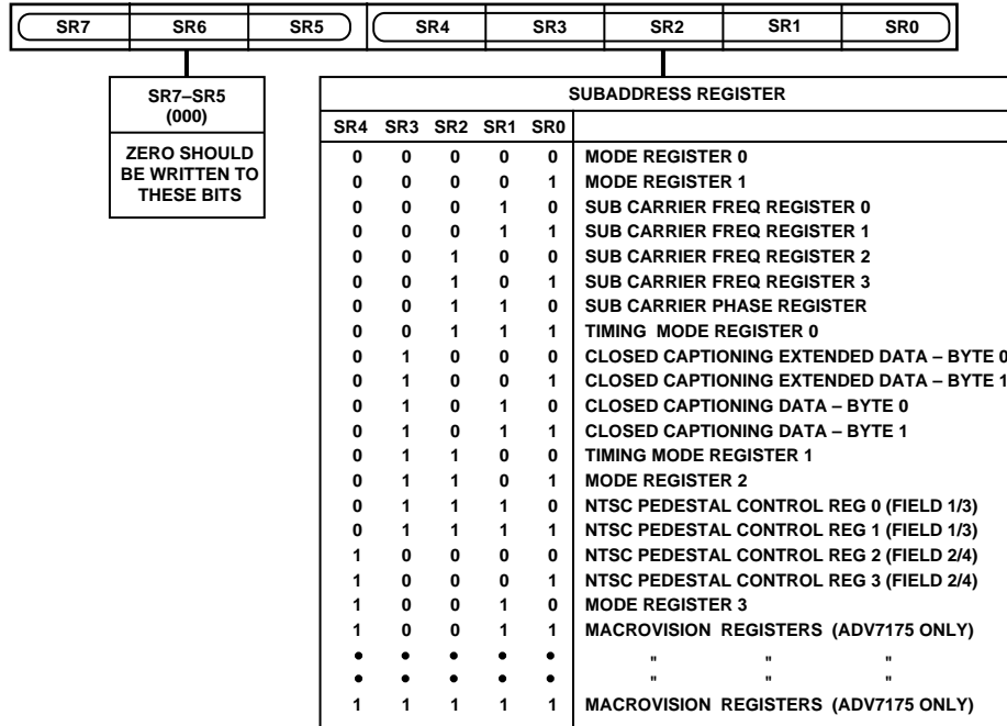
Figure 30. Subaddress Register
