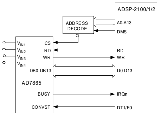
Figure 20. AD7865-ADSP-2100 Interface
